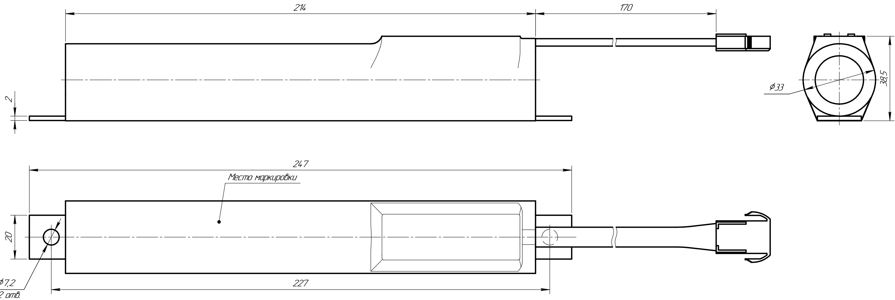
Батарея 9,6 В 6000 мАч
