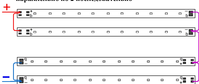
Включение 4-х модулей без разъема по схеме: 2 группы параллельно по 2 последовательно
