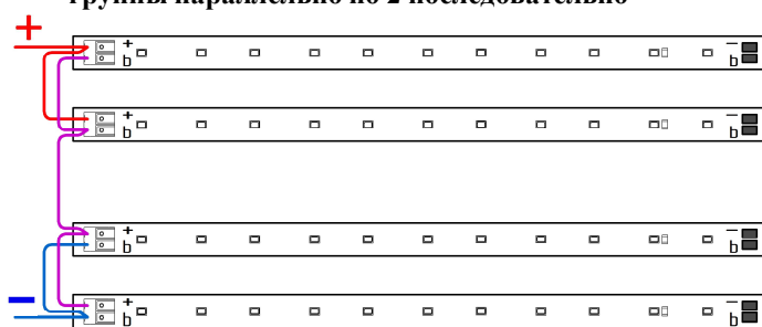
Включение 4-х модулей с разъемом DL250 по схеме: 2 группы параллельно по 2 последовательно
