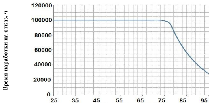
Зависимость времени наработки ИПС на отказ от температуры
