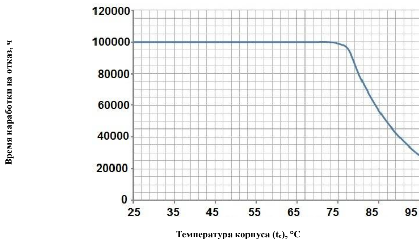
Зависимость времени наработки ИПС на отказ от температуры
