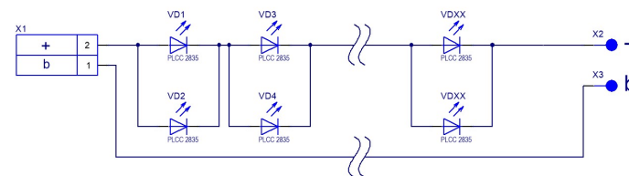
Исполнение модуля без разъема LINE 470x11.6 AL1 SxP Lumileds 2835
