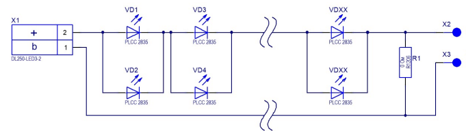
Исполнение модуля с разъемом LINE 470x11.6 AL1 SxP Lumileds 2835 DL250
